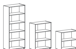
iHC 85 850 x 430 x 1930 iMC 85 850 x 430 x 1165 TLC 85 850 x 430 x 795
